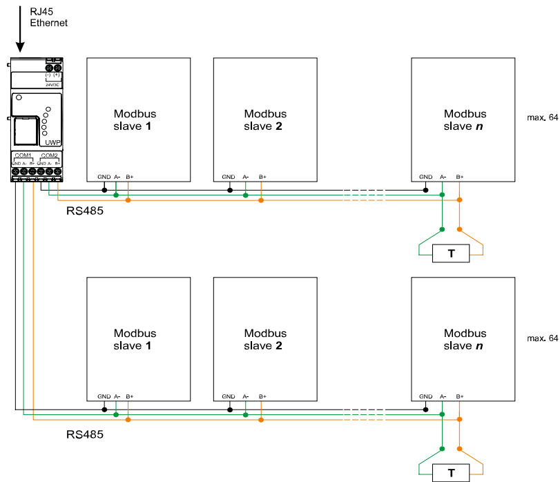
Fig. 1 Modbus-RTU-Verbindungsschema. COM 1 Master, COM 2 Master
